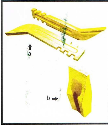
a: Shank Part No: 9F 5124 b: Tip Part No: 2D 5572
